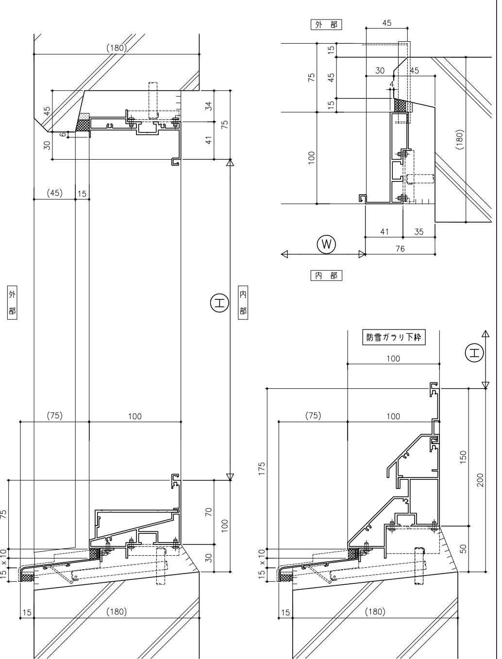
アゴ付納まり S:1/6
